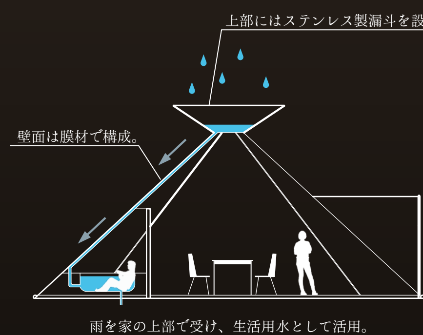
住戸断面 (s=1/250)
