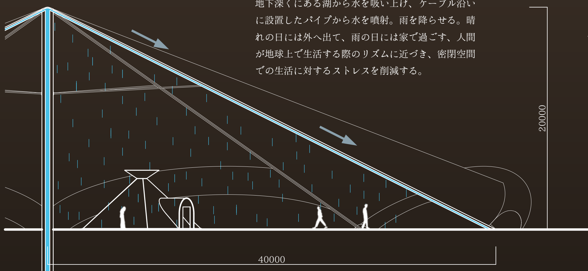
断面図 (s=1/500)
