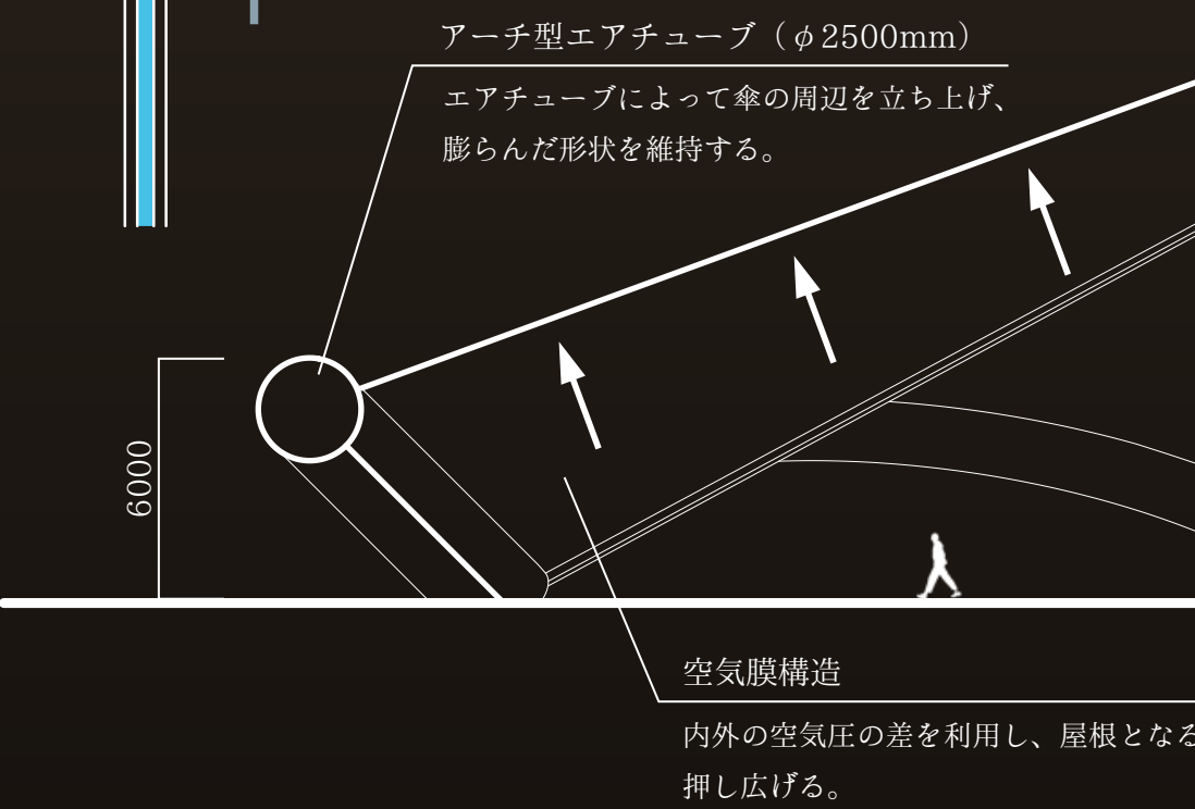
断面図 (s=1/500)
